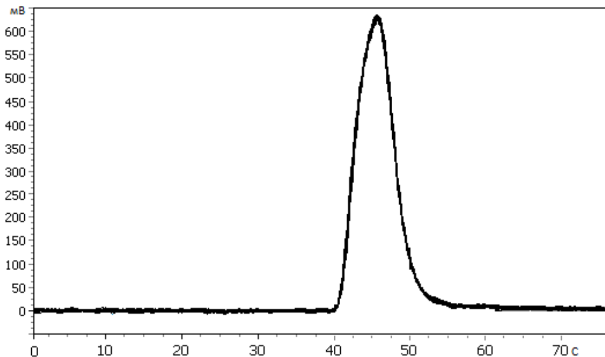
Рисунок Г.1 – Типовой пик ОС в пробе ПГ на УФ-флуоресцентном анализаторе
