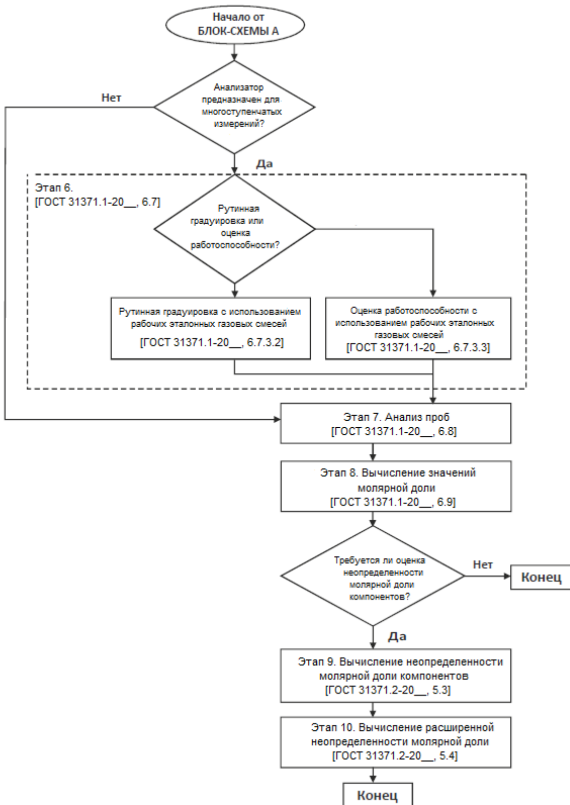
Рисунок 2 – Процедуры определения молярной доли и неопределенности — этапы с 6 по 10
